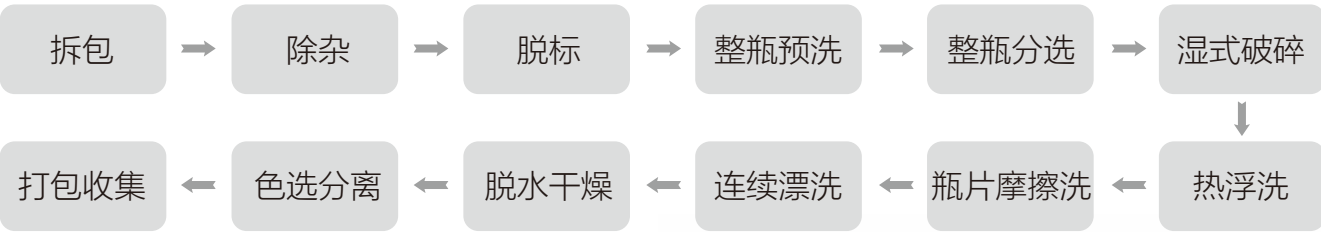
化纤级洗瓶线工艺流程
